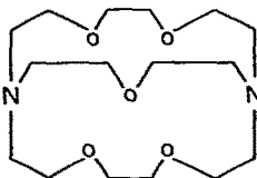
Kryptofix 221 Na +
