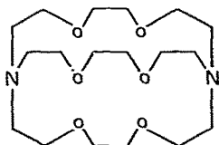
Kryptofix 222 K +
