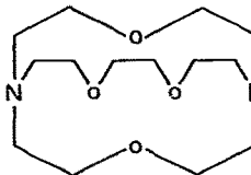
Kryptofix 211 Li +
